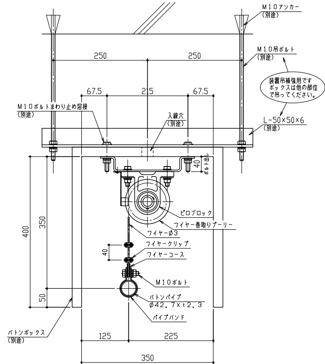
A-A断面図 S=1/5
