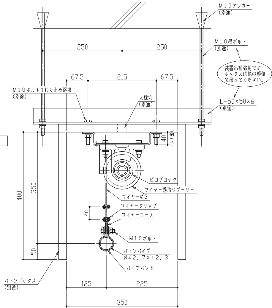
A-A断面図 S=1/5
