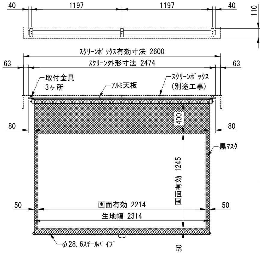
外観図 1/30
