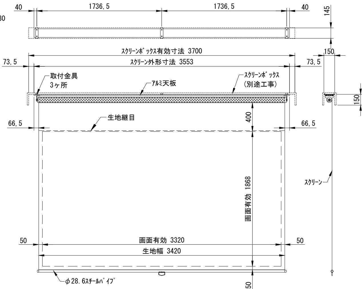
断面図 1/30
