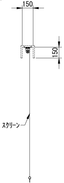
断面図 1/30
