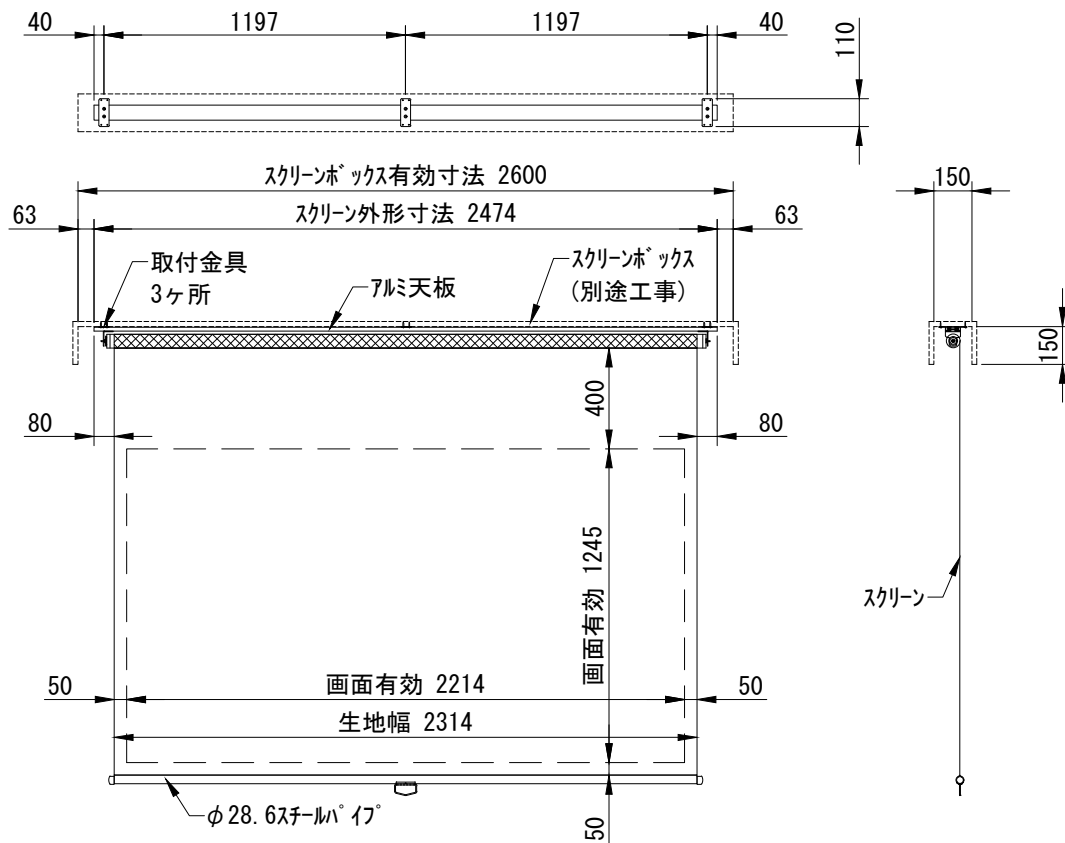
断面図 1/30
