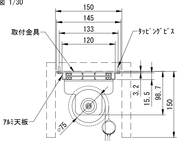
外観図 1/30
