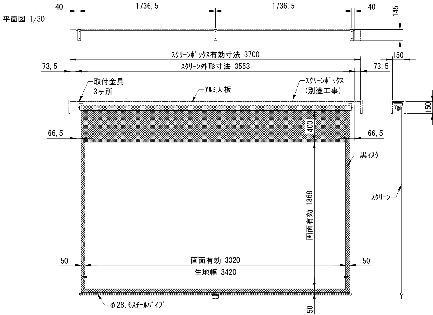
断面図 1/30
