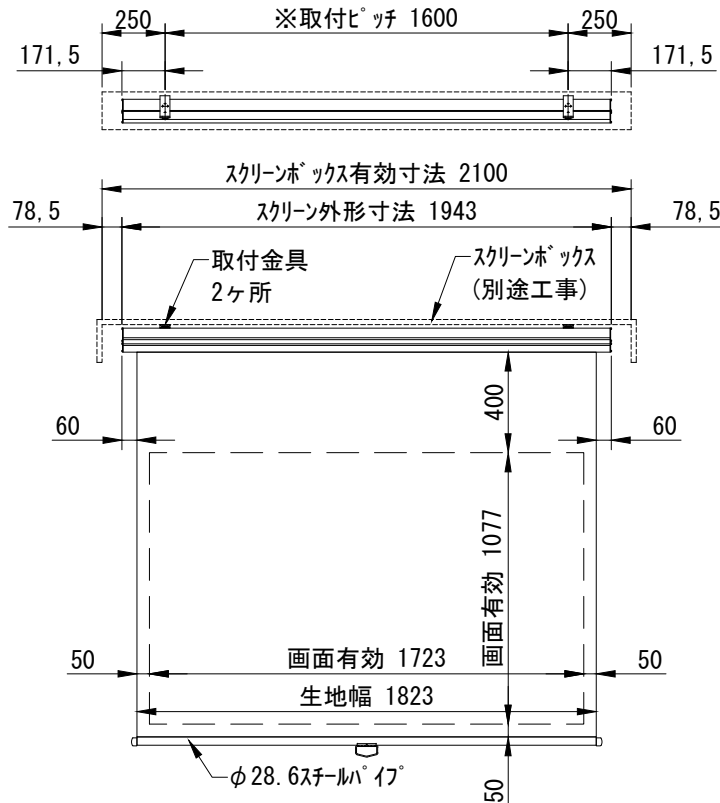
外観図 1/30
