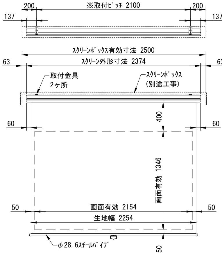
外観図 1/30
