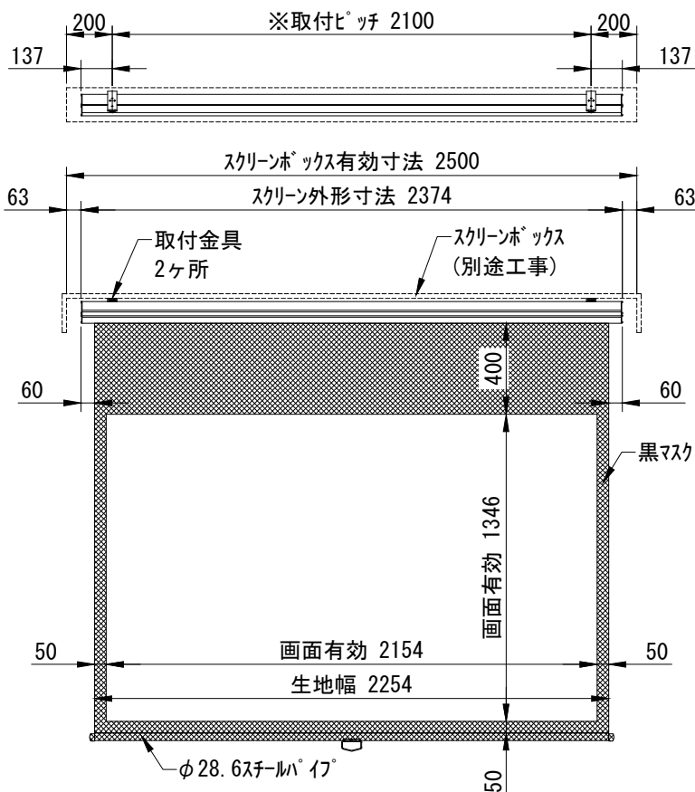
外観図 1/30
