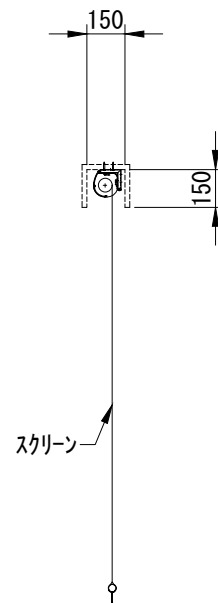
断面図 1/30
