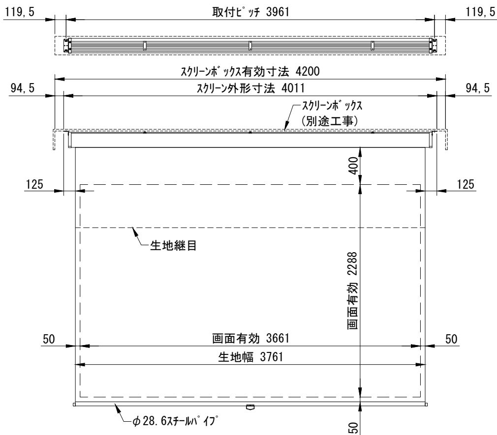
外観図 1/40
