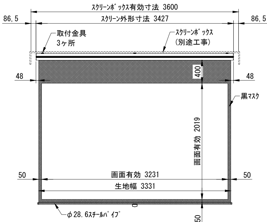
外観図 1/40
