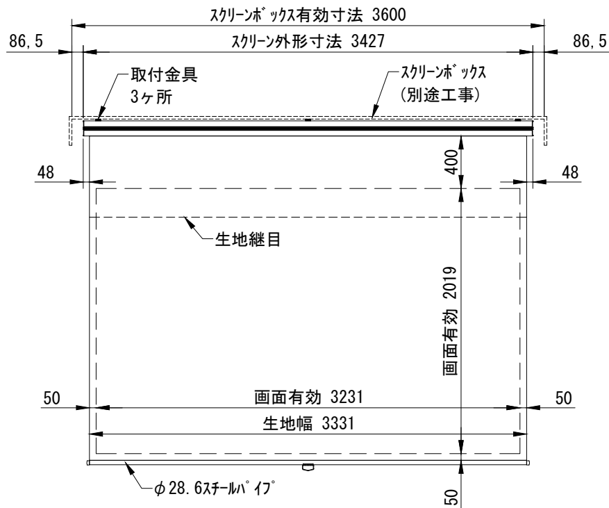
外観図 1/40
