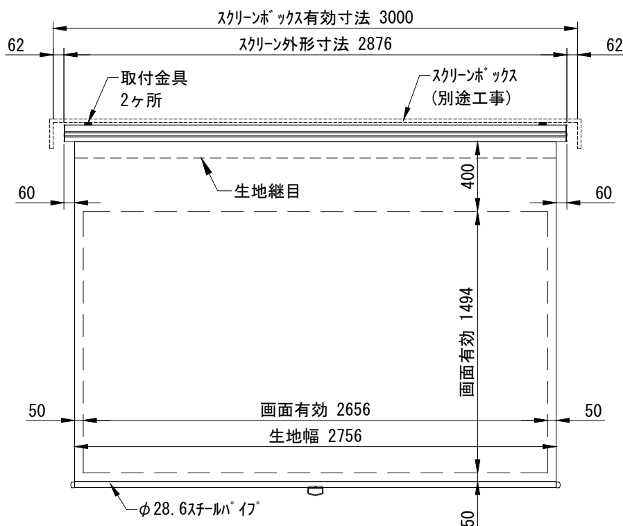
外観図 1/30
