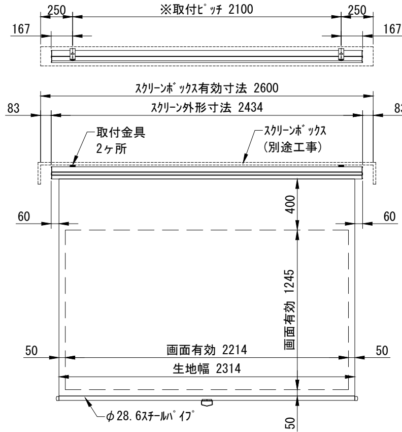
外観図 1/30
