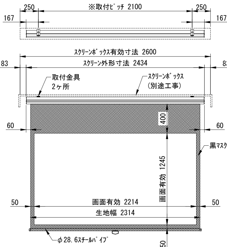
外観図 1/30
