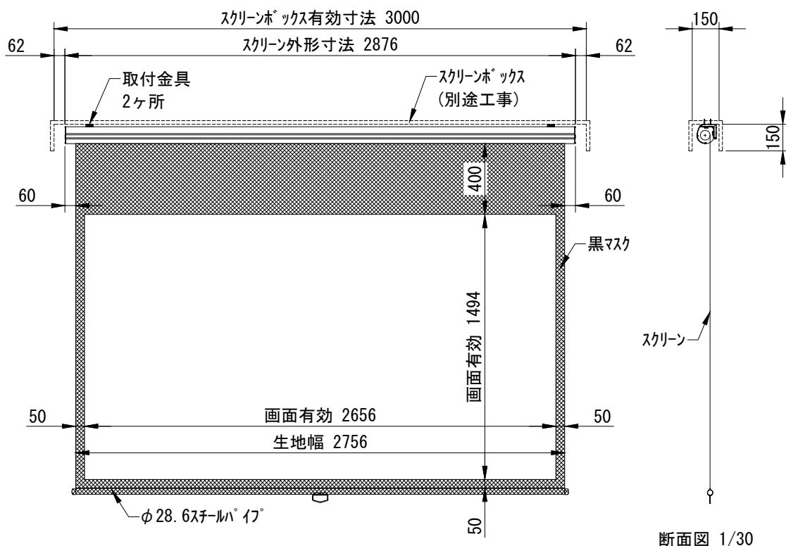
外観図 1/30
