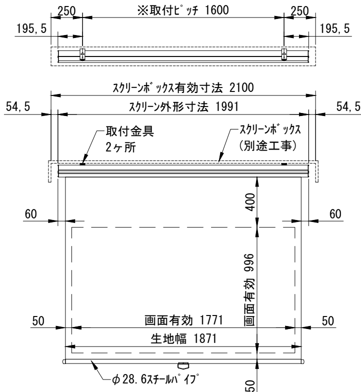
外観図 1/30
