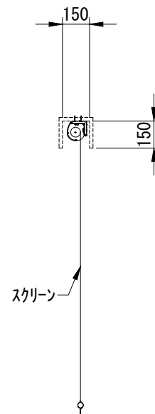
断面図 1/30
