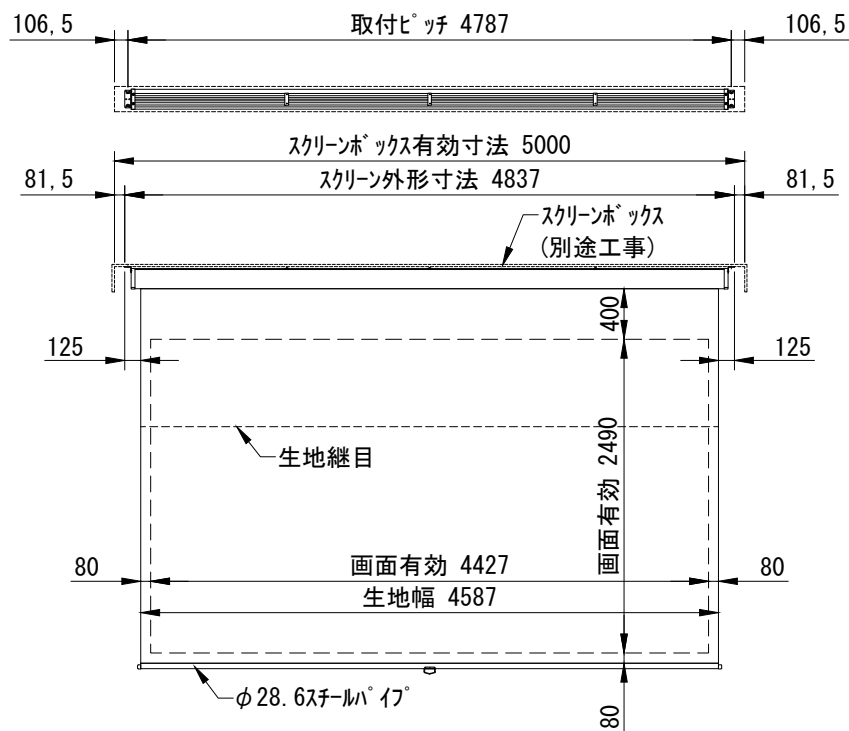
外観図 1/60
