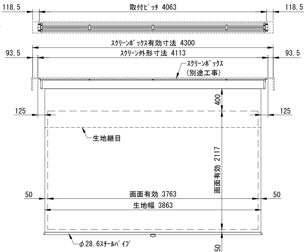
外観図 1/40
