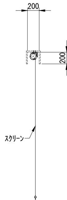
断面図 1/40
