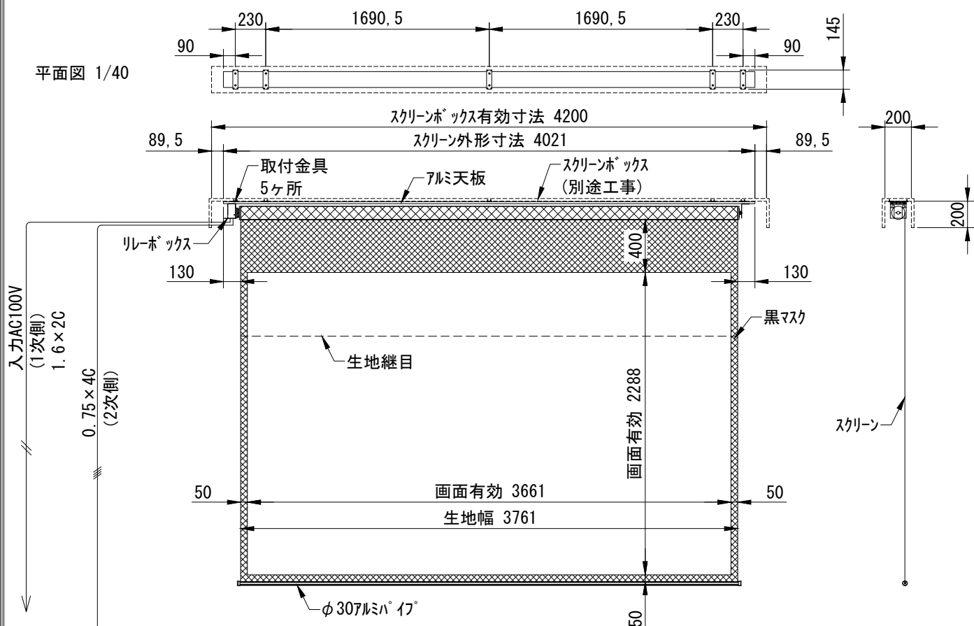
外観図 1/40
