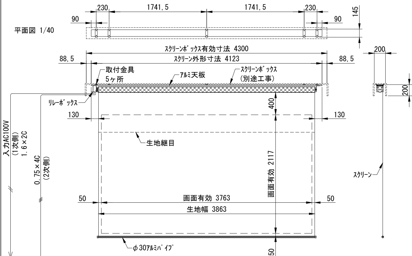
外観図 1/40
