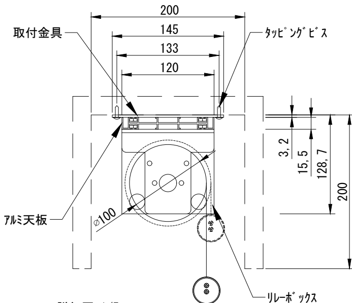
詳細図 1/5
