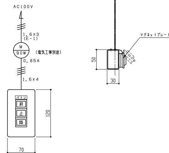
操作スイッチ及び電気系統図
