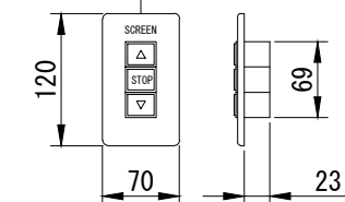
1連用フルカラー埋込み型スイッチ
