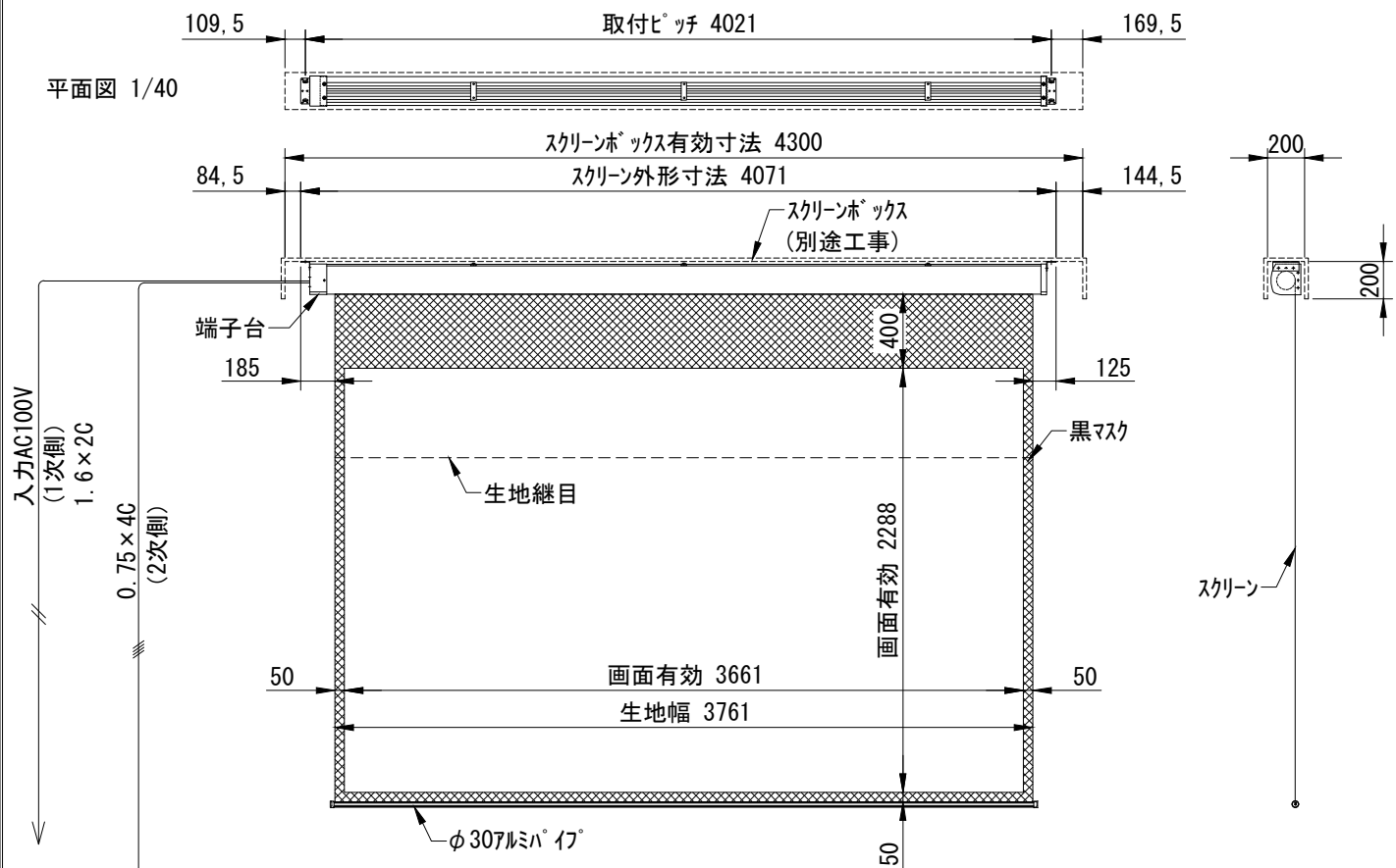
外観図 1/40
