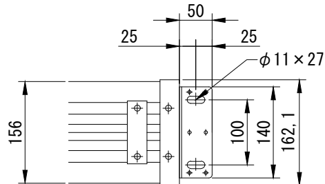
外観図 1/40
