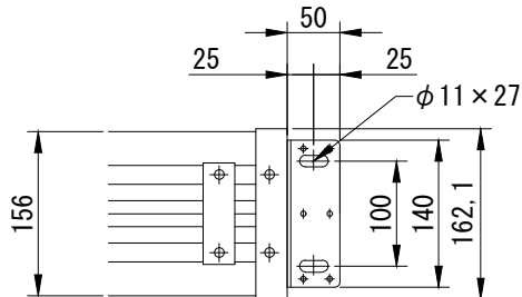
外観図 1/40
