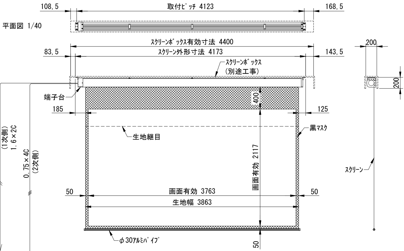
外観図 1/40
