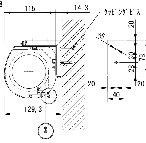
壁面取付時 1/5
