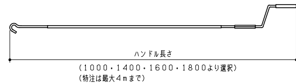
操作ハンドル
