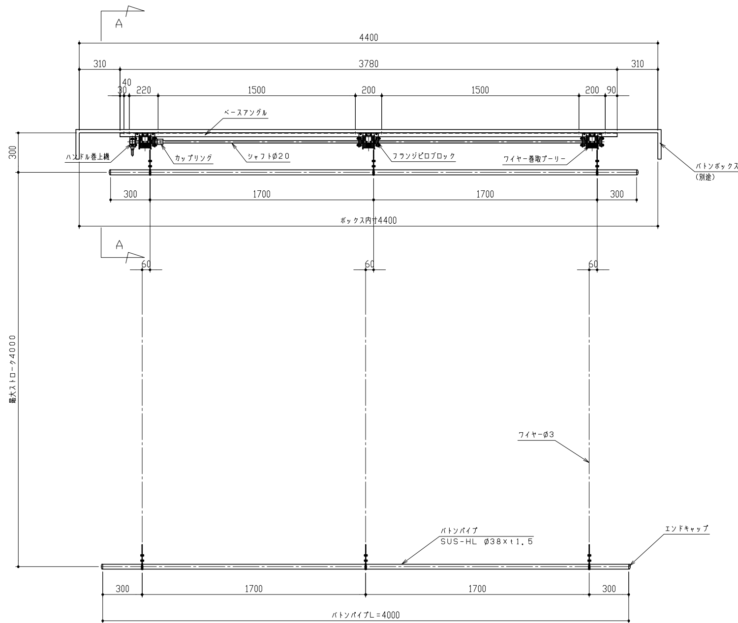
正面図 S=1/20
