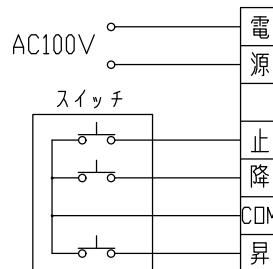
結線図
