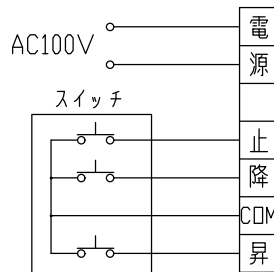
結線図
